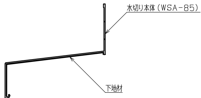
A-A断面図
