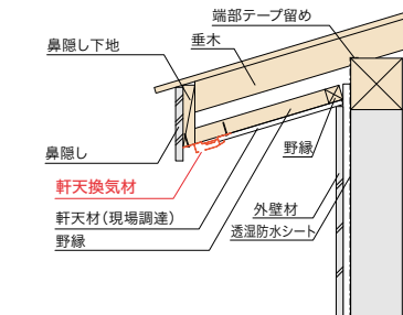
参考納まり図
