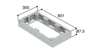
BU-CUB-8060-HB1 アジャスター 1 段
