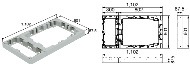
CUB-8060-H1 アジャスター 1 段
