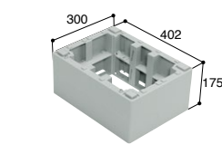
BU-CUB-6040-HD2 アジャスター 2 段
