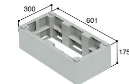
BU-CUB-8060-HB2 アジャスター 2 段
