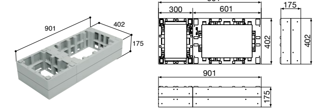
CUB-6040-H2 アジャスター 2 段
