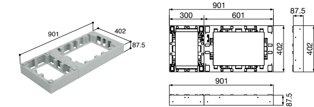
CUB-6040-H1 アジャスター 1 段
