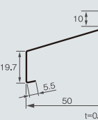
WCF-S50寸法図
