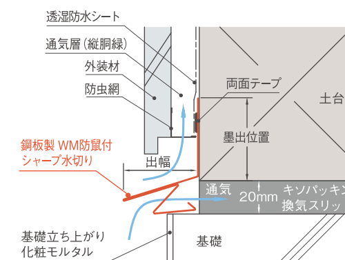
参考納まり図
