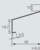
WCF-S45寸法図
