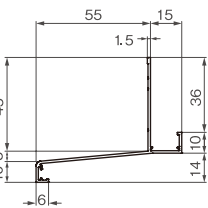
HA-55-L27 (出幅55mm) 寸法図
