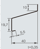
WCF-S40寸法図
