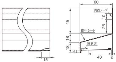
寸法図
