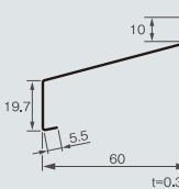
WCF-S60寸法図
