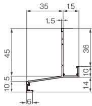
HA-35-L27 (出幅35mm) 寸法図
