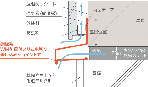
参考納まり図
