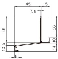
HA-45-L27 (出幅45mm) 寸法図
