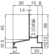
HKA-30-L27 (出幅30mm) 寸法図
