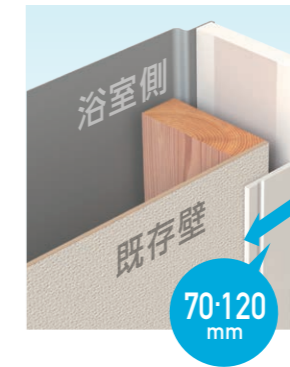
抗菌樹脂枠 隙間化粧カバー ムクタイプ
