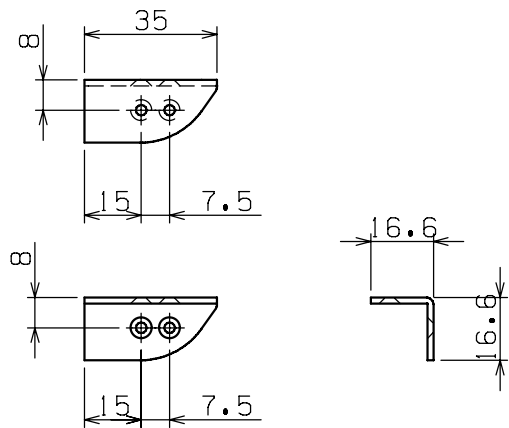
NR-1S05用棚板受金具
