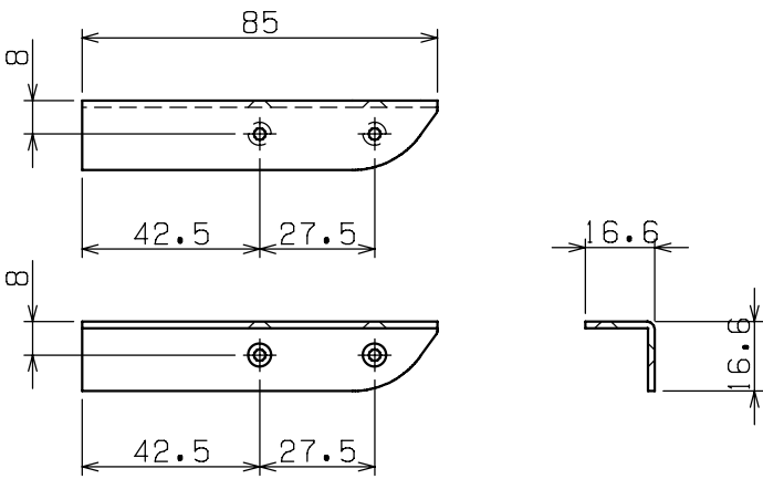
NR-IS10用棚板受金具
