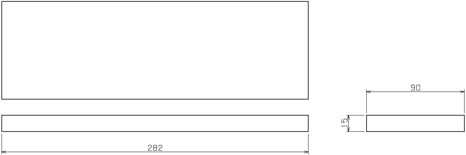
NR-303010/NR304510/NR-306010用棚板
