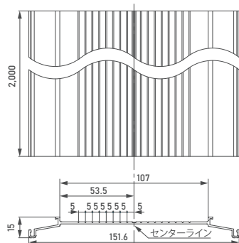
寸法図
