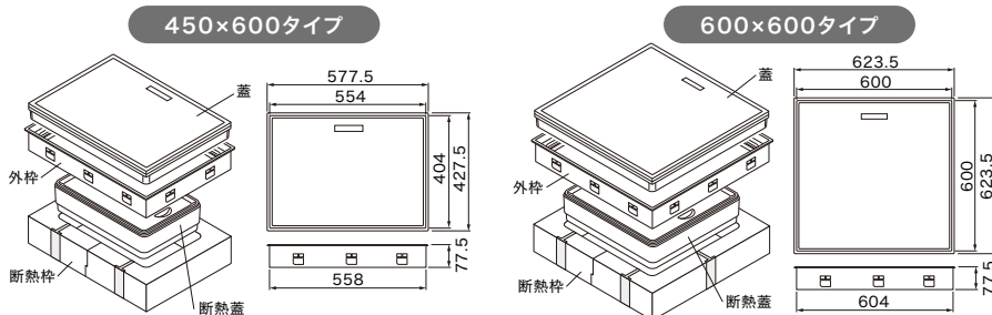
寸法図
