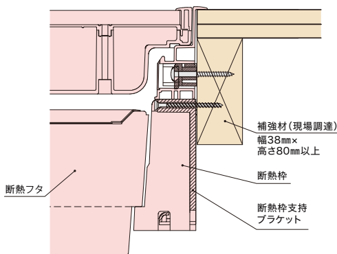
標準納まり図 (SPF-R60F12-UB3の場合)
