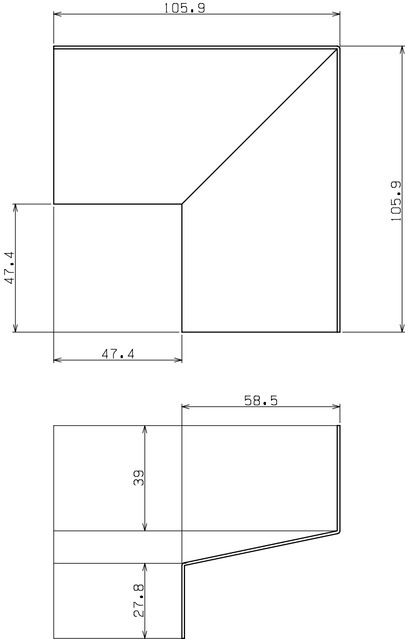
入隅部カバー部材
