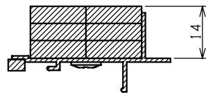
断面図A-A (1/1)
