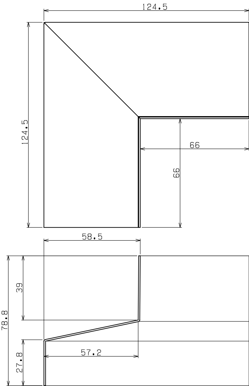
出隅部カバー部材
