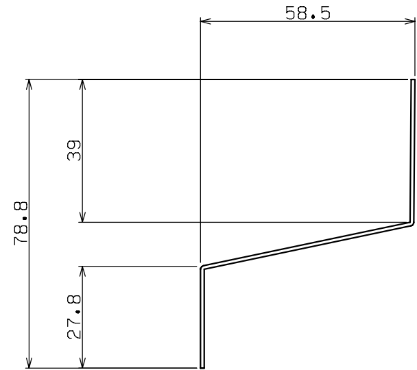
浸水対策水切り エンド部カバー部材
