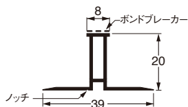
参考納まり図
