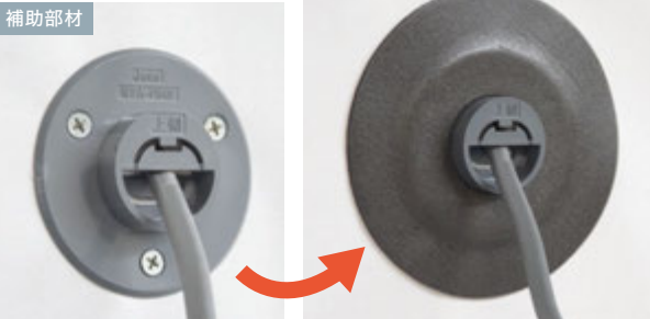
防水役物 配管用 WPA-P40との併用
